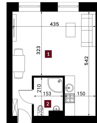
Schemat kondygnacji
