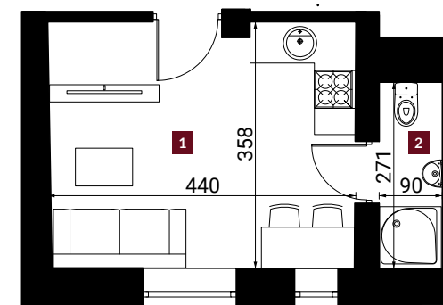
Rzut lokalu
