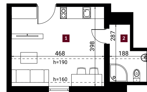
Rzut lokalu
