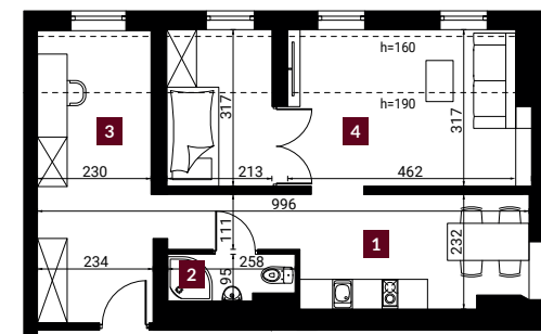
Rzut lokalu
