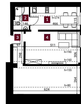
Schemat kondygnacji
