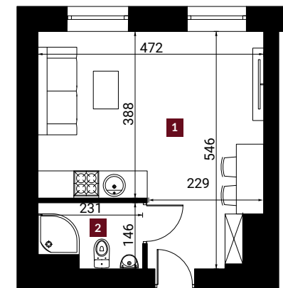
Rzut lokalu
