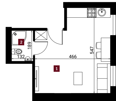
Rzut lokalu
