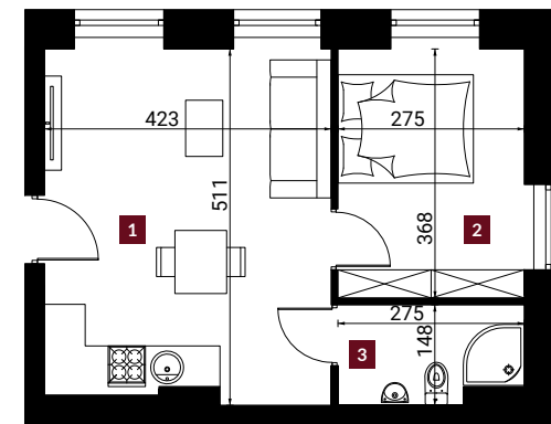
Rzut lokalu
